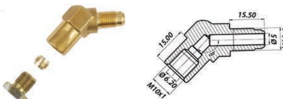
Dirsek Takımı 135° M10x1 / M10x1 Elbow Set 135° M10x1 / M10x1
