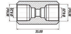
Boru Birleştirici Takım Ø8 - Ø8 Pipe Coupling Set Ø8 - Ø8
