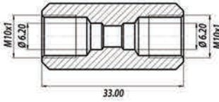
Boru Birleştirici Takım Ø6 - Ø6 Pipe Coupling Set Ø6 - Ø6
