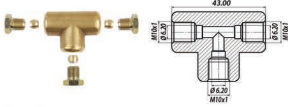
T Takım Ø6 x Ø6 x Ø6 T Set Ø6 x Ø6 x Ø6
