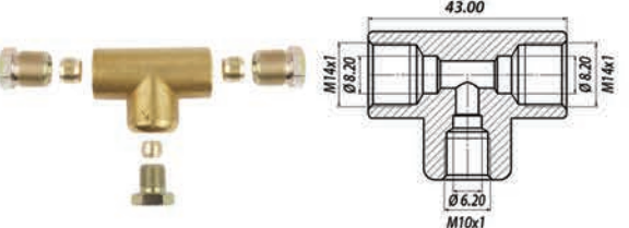
T Takım Ø8 x Ø6 x Ø8 T Set Ø8 x Ø6 x Ø8
