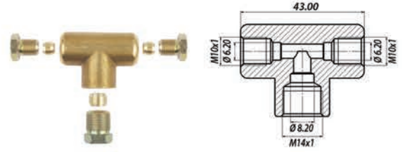
T Takım Ø6 x Ø8 x Ø6 T Set Ø6 x Ø8 x Ø6
