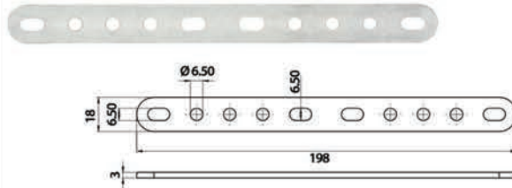
Bağlantı Sacı Uzun 200 x 18 x 3,00 mm Connection Steel Long 200 x 18 x 3,00 mm
