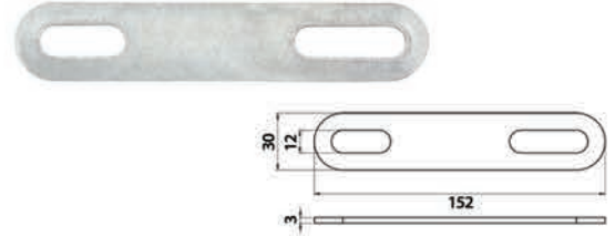
Bağlantı Sacı 152 x 30 x 3,00 mm Connection Steel 152 x 30 x 3,00 mm
