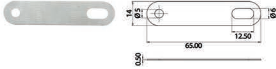
Bakır Boru Kroşe 65,00 x 14,00 x 0,50 mm Copper Pipe Clamp 65,00 x 14,00 x 0,50 mm
