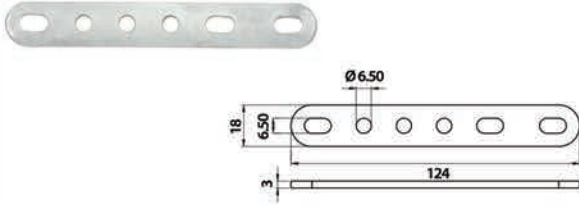
Bağlantı Sacı Kısa 124 x 18 x 3,00 mm Connection Steel Short 124 x 18 x 3,00 mm
