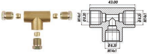
T Takım Ø8 x Ø8 x Ø8 T Set Ø8 x Ø8 x Ø8
