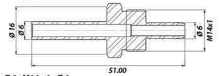
Termoplastik Rakor Ø6 - M14x1 - Ø6 Thermoplastic Bolt Ø6 - M14x1 - Ø6
