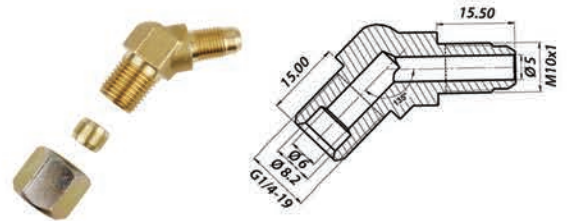
Dirsek Takımı 135° M10x1 / G1/4-19 Elbow Set 135° M10x1 / G1/4-19
