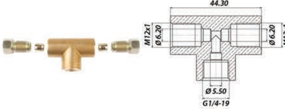
CNG Manometre T Takım CNG Manometer T Set
