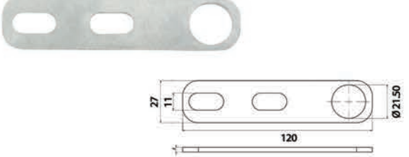
Bağlantı Sacı CNG 01 Connection Steel CNG 01
