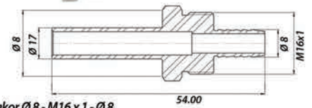
Termoplastik Rakor Ø8 - M16x1 - Ø8 Thermoplastic Bolt Ø8 - M16x1 - Ø8
